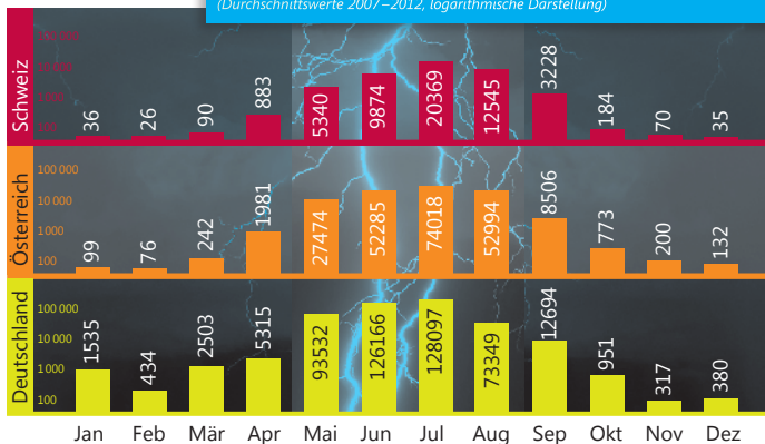
Statistik der Blitze in Deutschland, Österreich und der Schweiz (Durchschnittswerte 2007 – 2012, logarithmische Darstellung)
